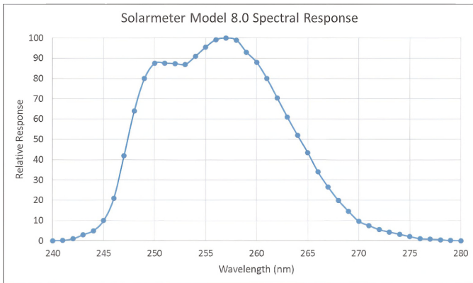
図1. モデル8.0のスペクトル応答
